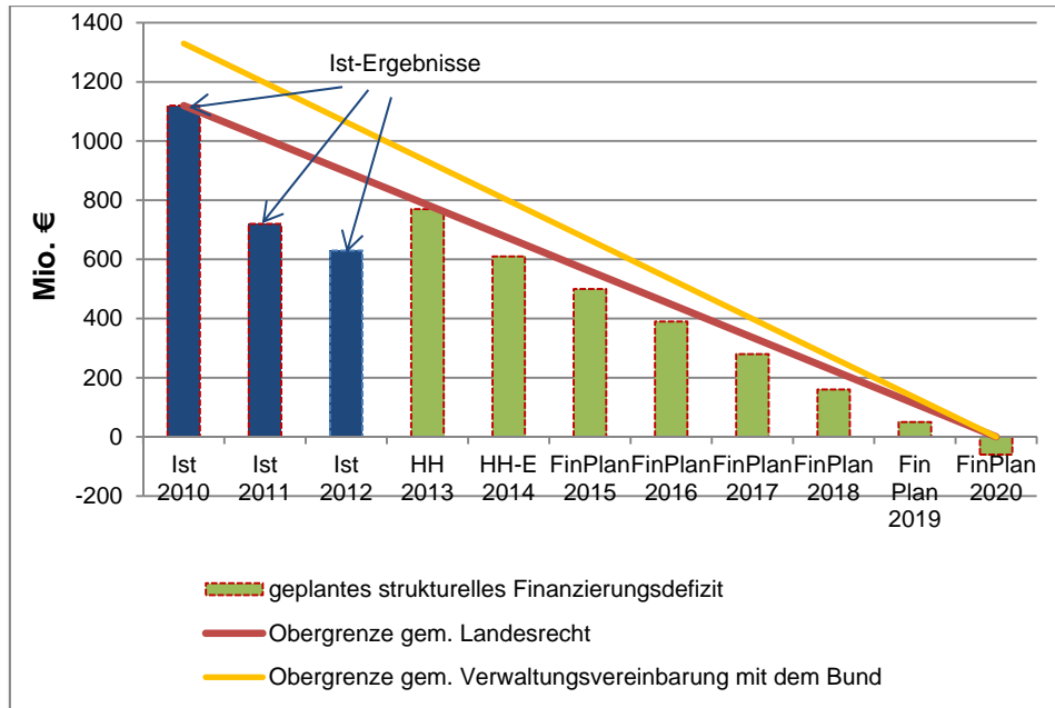
Abbildung 1: Zulässige Obergrenze und tatsächlicher Abbau des strukturellen Finanzierungsdefizits bis 2020
